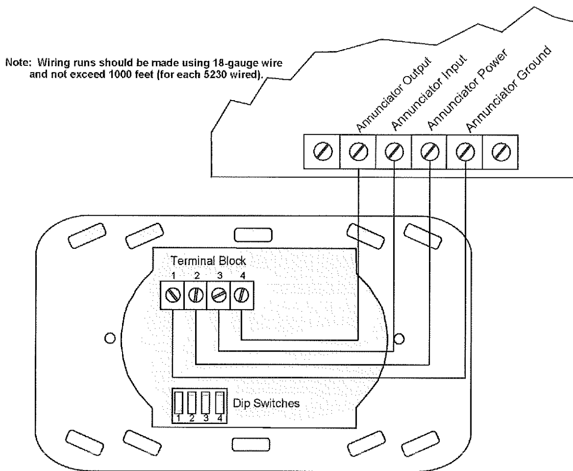
Wiring the 5230
