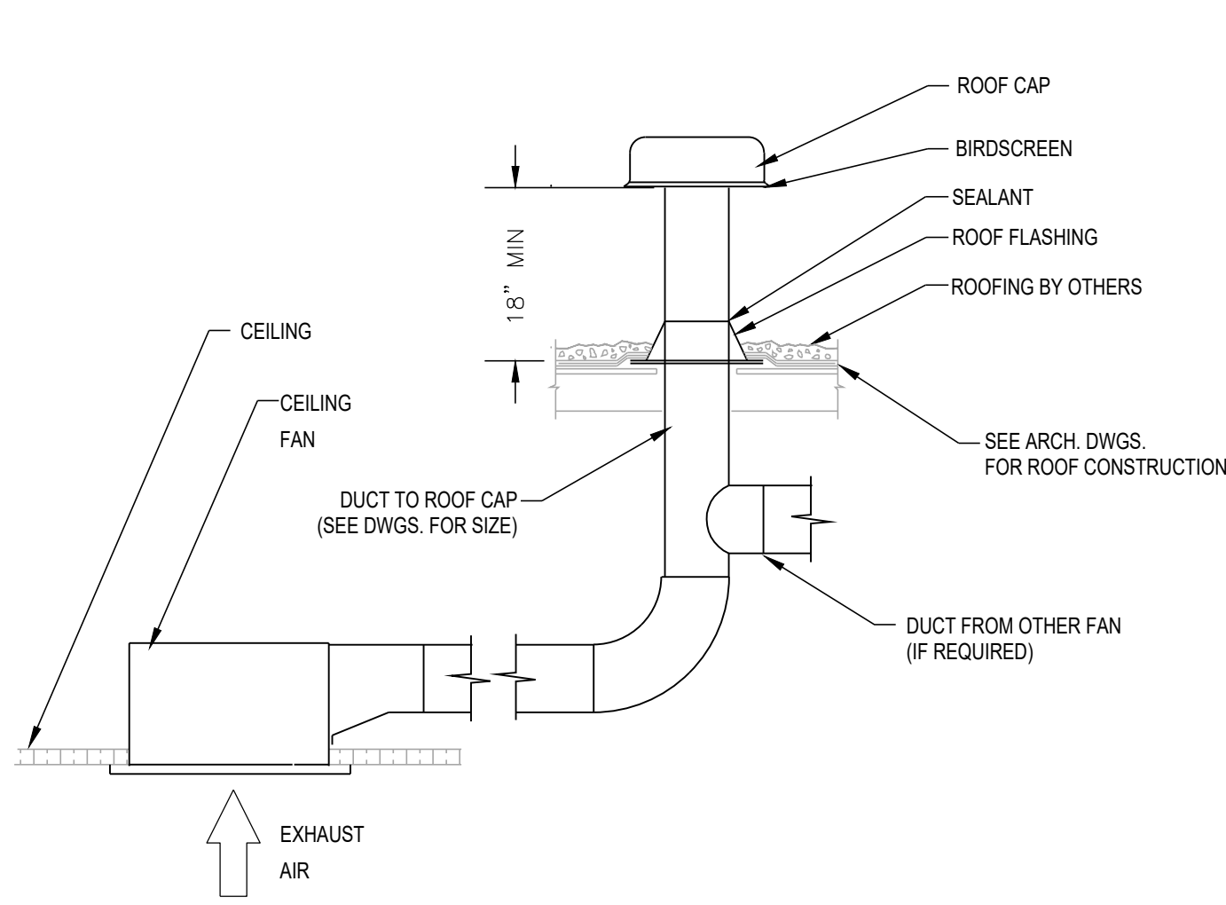
A RESTROOM EXHAUST FAN DETAIL NTS
